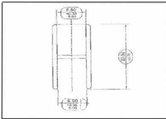
T014C Hトリミング 6.50mm
