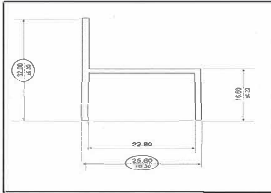
T014B hトリミング 22.80mm
