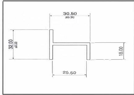
T013 hトリミング 25.50mm
