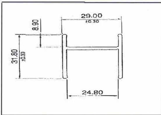
T014B Hトリミング 24.80mm
