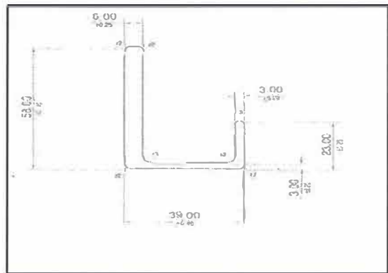
T021 ハッチプロファイル
